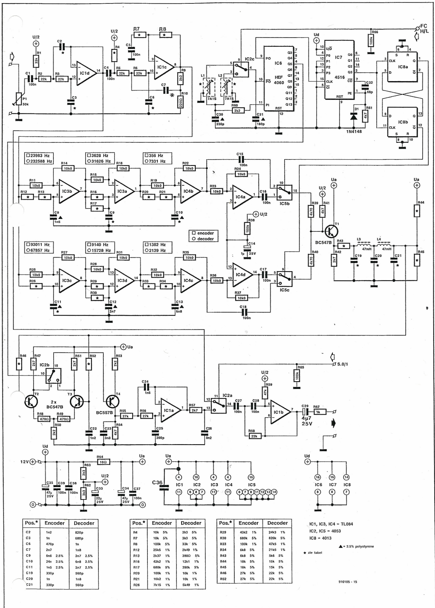
Figuur 5. Het schema van zowel de scrambler- als de descrambler-schakeling.
